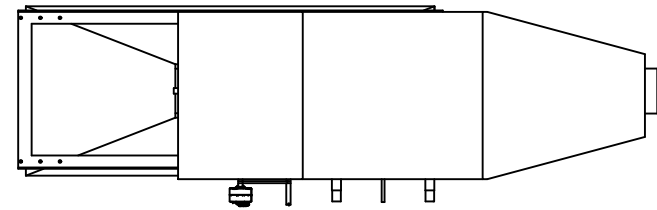
C65HPNG DualMode WT6080 Wasseranschluß rechts Abgasausgang nach hinten
